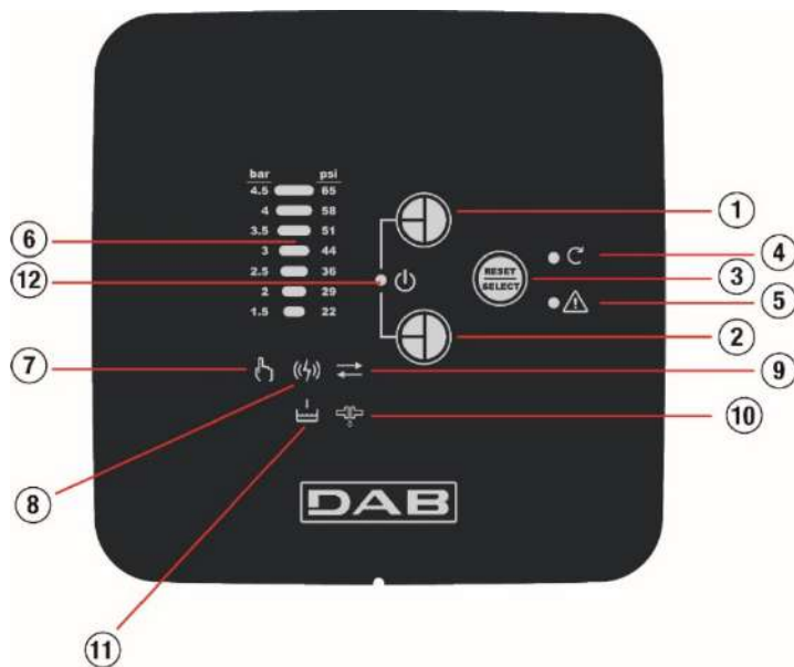
12. kép: COM BOX szerkezeti egység panelje
