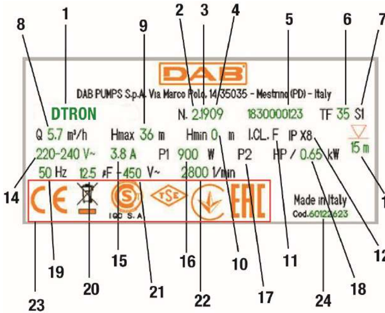
Kuva 4 Arvokilpi
